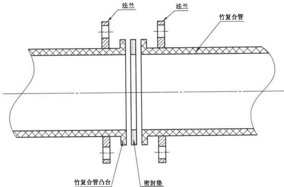
图 D.1 法兰连接组装图
